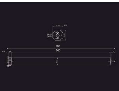
El motor vía radio más corto del mundo con solo 29.6 cm
