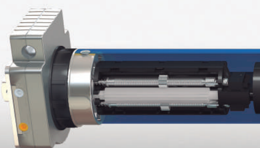
Alta potencia, Motor de hasta 140 newtons
